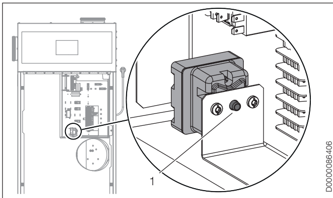
1 Rückstellknopf Sicherheitstemperaturbegrenzer
