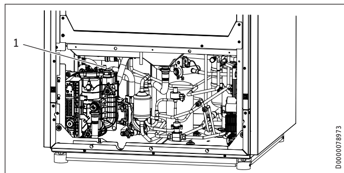
1 Entlüftungsventil
