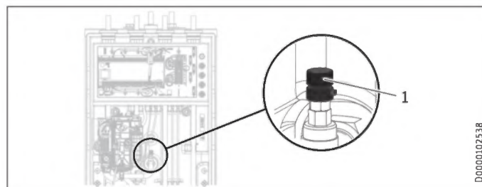
1 Entlüftungsventil
