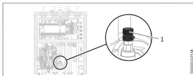
1 Ontluchtingsventiel
